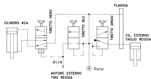
SCHEMA PNEUMATICO PNEUMATIC CHART
